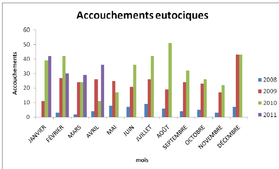
Graphique 3.2 Dynamique des accouchements eutociques, Février 2008 – avril 2011
