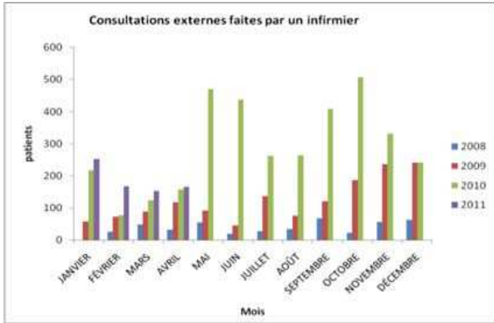
Graphique 2.2 : dynamique des consultations externes ou de triage faites par les infirmiers février 2008-avril 2011
